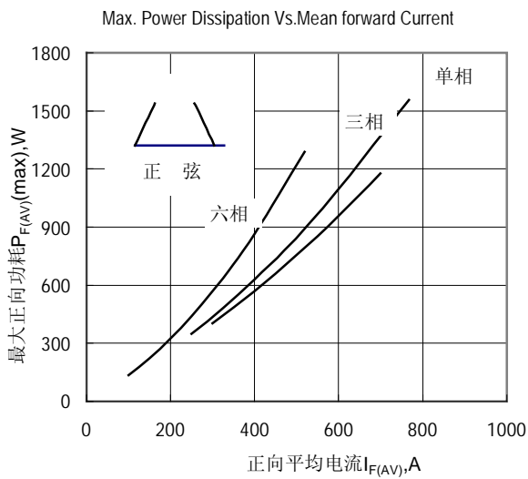
Fig.3 最大功耗与正向平均电流关系曲线
