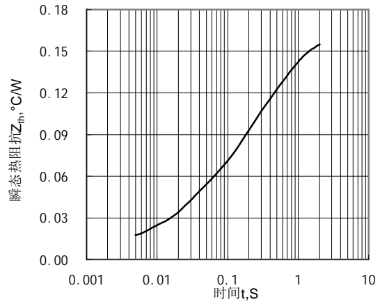
Fig.2 结至管壳瞬态热阻抗曲线
