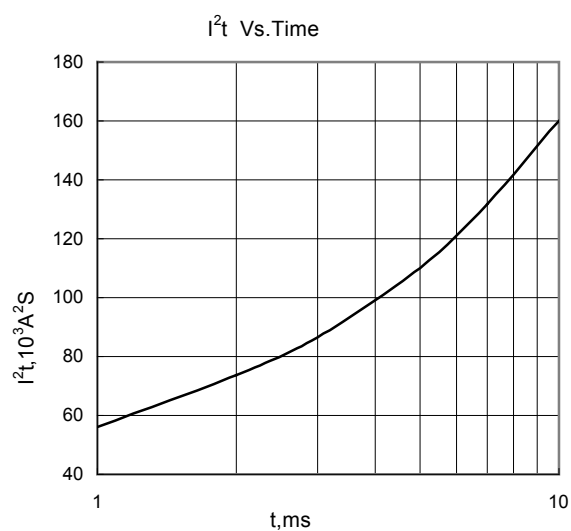
Fig.4 I^2t
