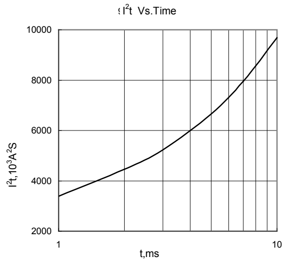
Fig.8 I^2t
